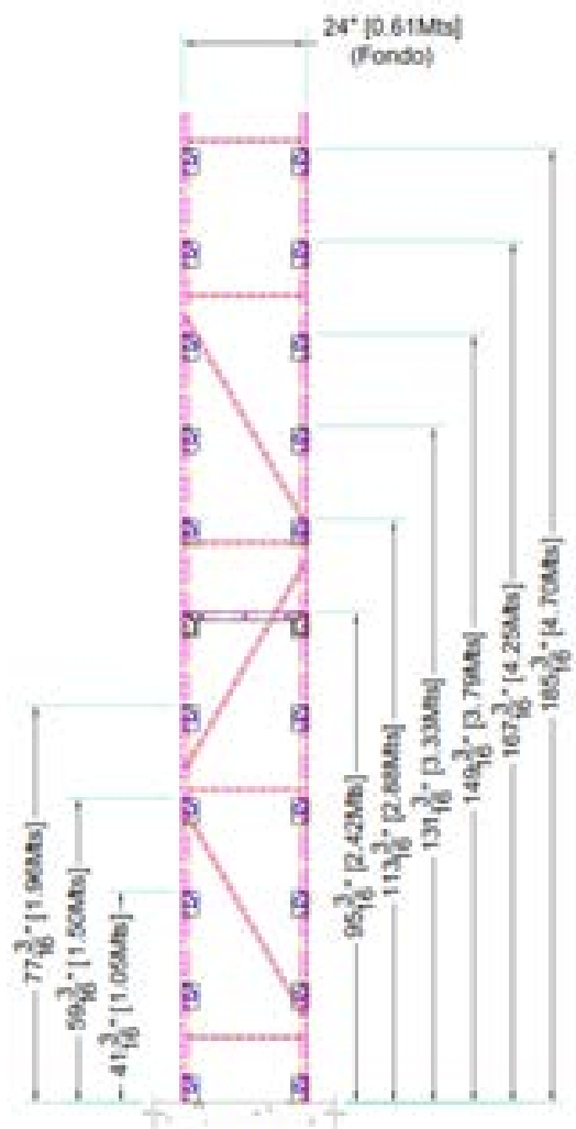
VISTA LATERAL DIRECHA
